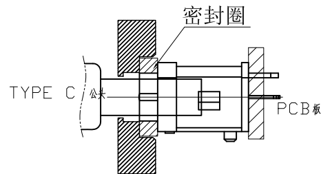
组装示意图
