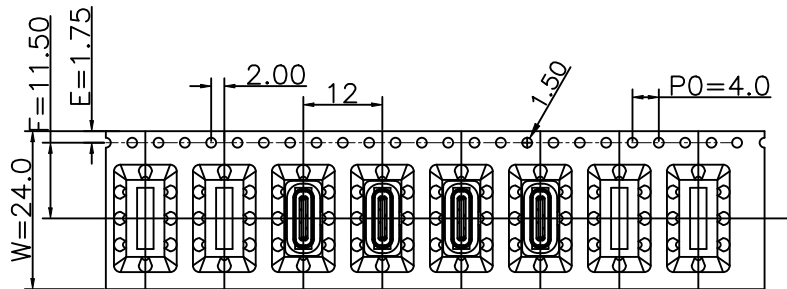
① 产品入载带示意图
