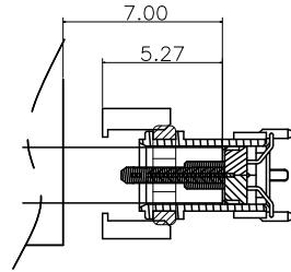
PLUG插入深度参考图
