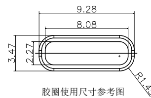
胶圈使用尺寸参考图
