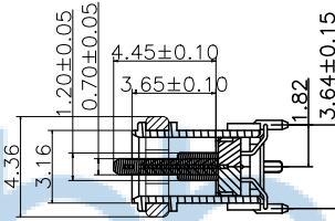
PLUG插入深度参考图
